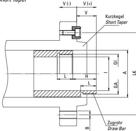
Ausführung 1: Kurzkegel Style 1: Short Taper
